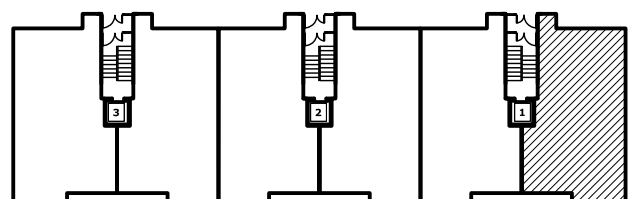
PLANTA BAJA BLOQUE "A" PORTAL 1 VIVIENDA "A" Superf Útil 52,29 m 2
