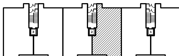
PLANTA BAJA BLOQUE "A" PORTAL 2 VIVIENDA "B" Superf Útil 52,30 m²
