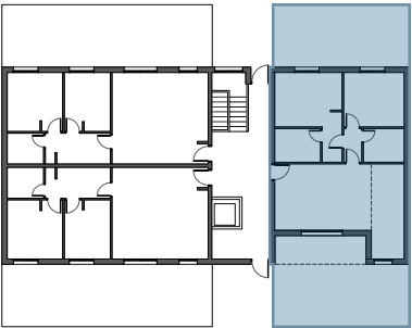
Bloque B_Planta baja
